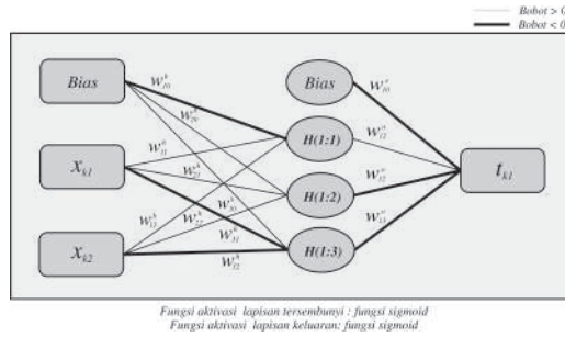
Gambar 2. Arsitektur Jaringan Saraf Tiruan
