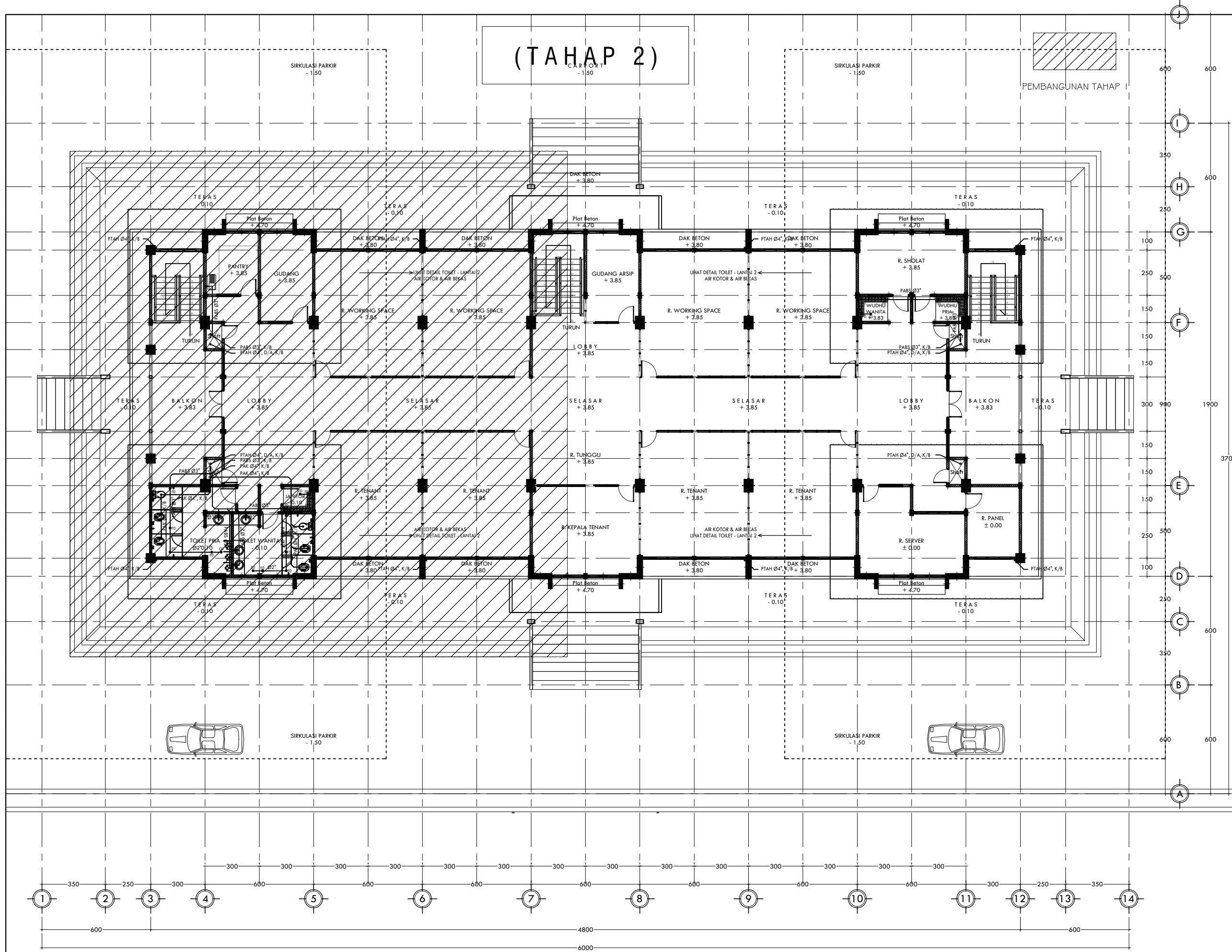
DENAH INSTALASI AIR KOTOR & AIR BEKAS LANTAI 2 SKALA 1 : 200
