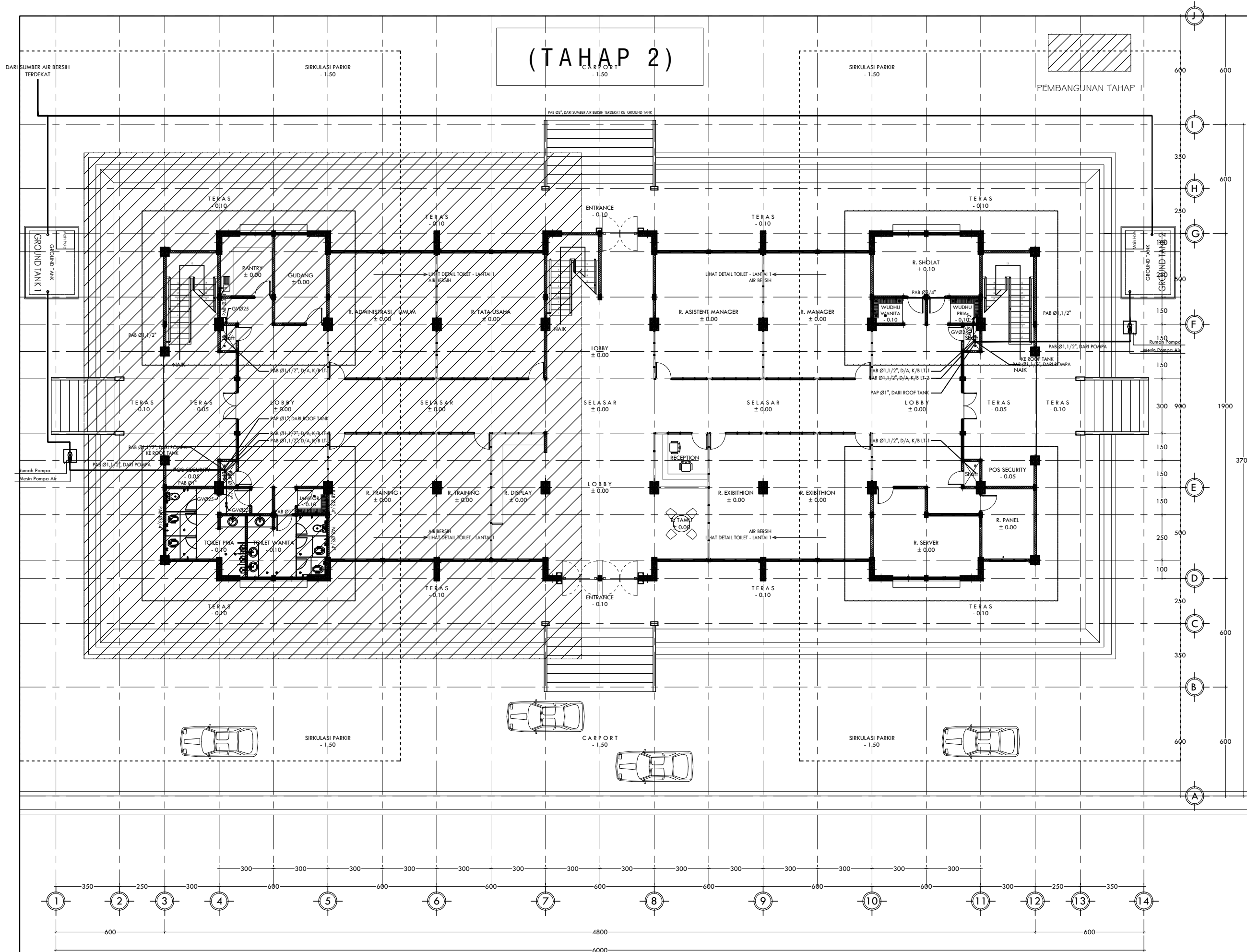
DENAH INSTALASI AIR BERSIH LANTAI I SKALA 1 : 200
