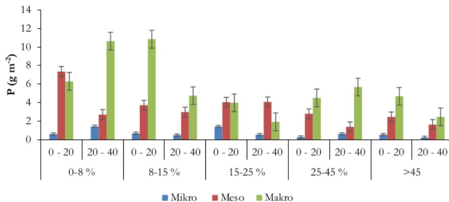
Gambar 1. Pasokan P per-kedalaman berdasarkan kemiringan lahan.
