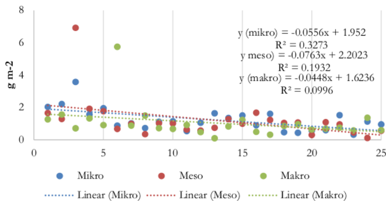
Gambar 2. Korelasi agregat tanah dengan pasokan P.
