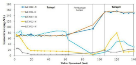
Gambar 4. Profil Perubahan Nitrogen Selama Start-up
