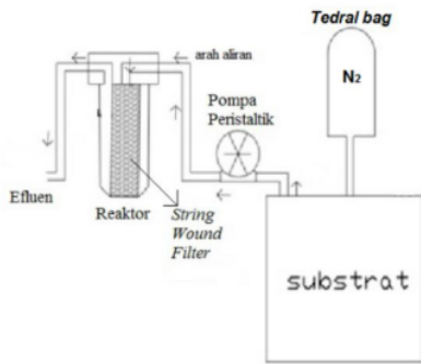
Gambar 3. Skema instalasi reaktor penelitian
