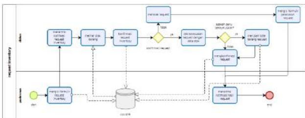
Gambar 5. Model bisnis permintaan barang yang diusulkan
