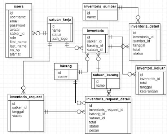
Gambar 8. Rancangan ERD
