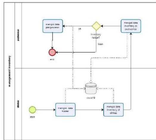
Gambar 6. Model bisnis pengendalian stok barang yang diusulkan
