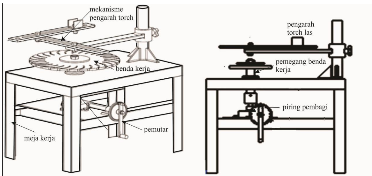
Gambar 6. Rancangan versi 1 dari perkakas bantu pegang dan pengarah untuk cakram pemutar
