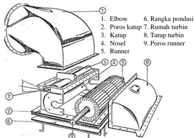
Gambar 1. Komponen-komponen pada turbin aliran silang ( cross-flow turbine ) [5]
