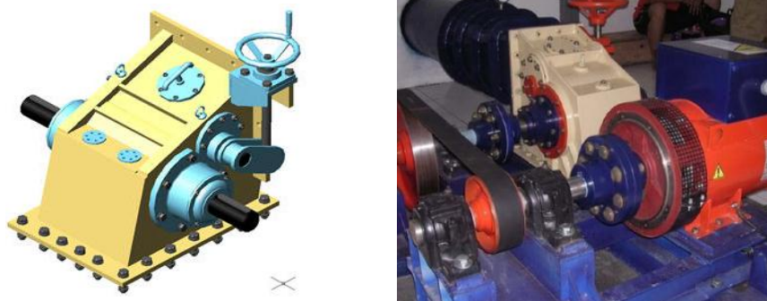
Gambar 2. Gambar turbin aliran silang tipe T14 (kiri) dan kondisi terpasang (kanan)[10]
