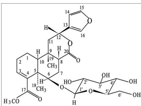
Gambar 2. Struktur Tinokrisposid
