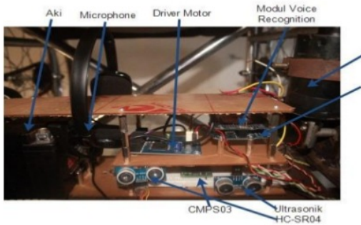
Gambar 4. Rangkaian Keseluruhan
