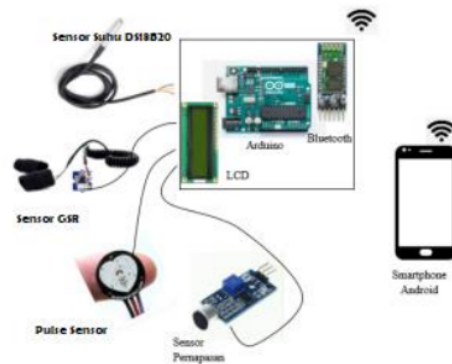
Gambar 1. Rancangan Perangkat Keras
