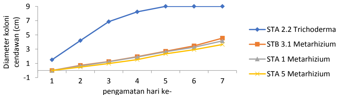
Gambar 2. Diameter koloni isolat cendawan entomopatogen setelah 1-7 hari inkubasi (Calibri 12, 1 spasi)
