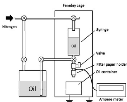
Fig.2. Mini static tester
