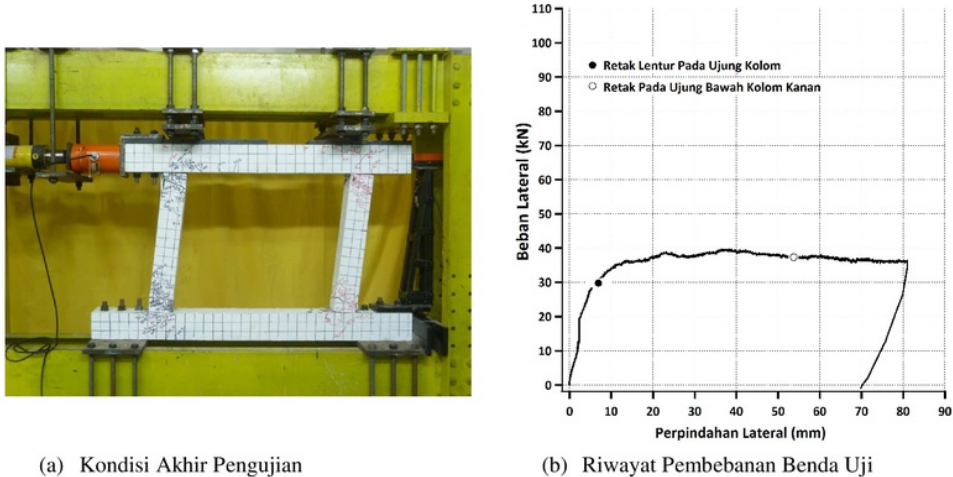
Gambar 5. Hasil Uji Benda Uji Struktur Portal Tanpa Dinding (BF)
