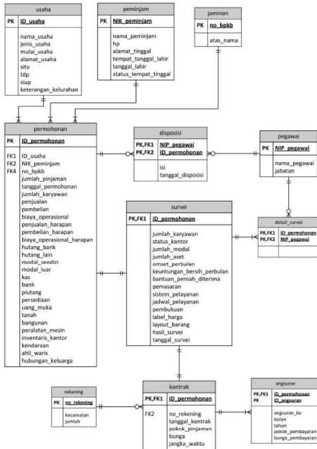
Gambar 4. ERD Sistem Informasi Permohonan Dana Bergilir
