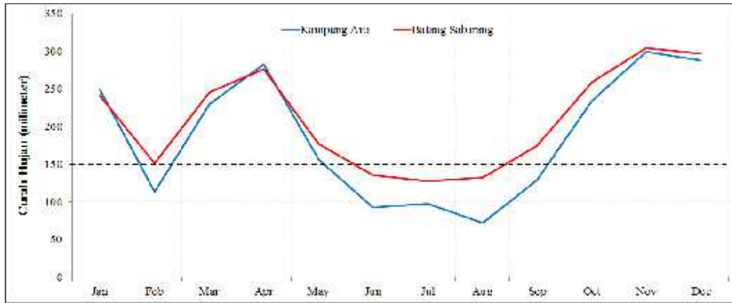
Gambar 15. Perbandingan curah hujan bulanan rata-rata di Kampung Aro dan Batang Sabarang pada periode tahun 1981-2015. Garis hitam putus-putus merupakan batasan awal musim kemarau (jika jumlah hujan < 150 mm/bulan) dan awal musim penghujan (jika jumlah hujan > 150 mm/bulan).
